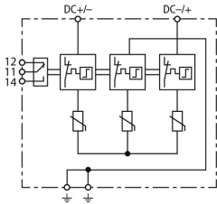
Prinzipschaltbild DCB YPV 1500 FM
