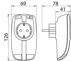
Maßbild DPRO 230 NT
