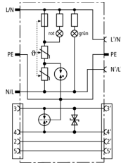
Prinzipialschaltbild DPRO 230 NT
